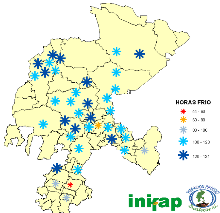
FIGURA 3. Horas frío acumuladas en la segunda decena del mes de enero del 2016.
