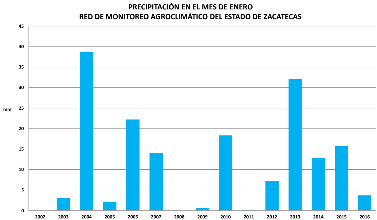
FIGURA 12. PRECIPITACIÓN PROMEDIO DEL MES DE ENERO, CONSIDERANDO LAS 36 ESTACIONES DE LA RED DE MONITOREO AGROCLIMÁTICO DEL ESTADO DE ZACATECAS.
