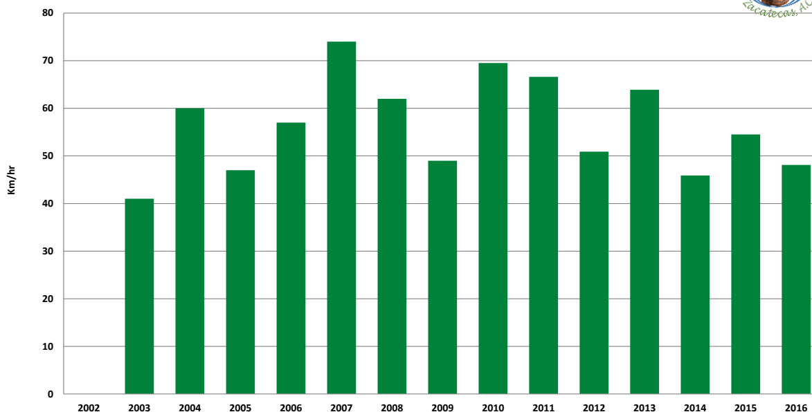
FIGURA 11. VALOR MÁXIMO DE VELOCIDAD DEL VIENTO EN EL MES DE ENERO, CONSIDERANDO LAS 36 ESTACIONES DE LA RED DE MONITOREO AGROCLIMÁTICO DEL ESTADO DE ZACATECAS.
