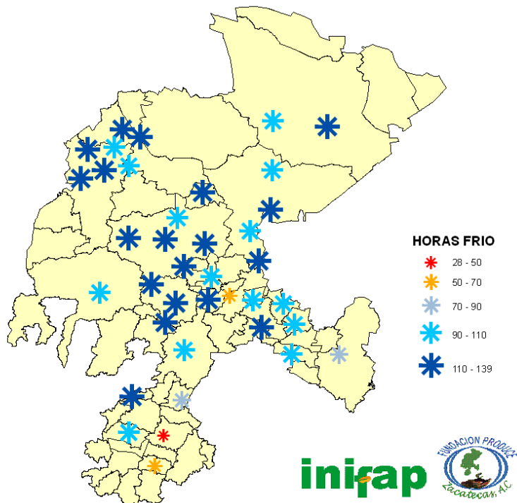
FIGURA 4. Horas frío acumuladas en la tercera decena del mes de enero del 2016.
