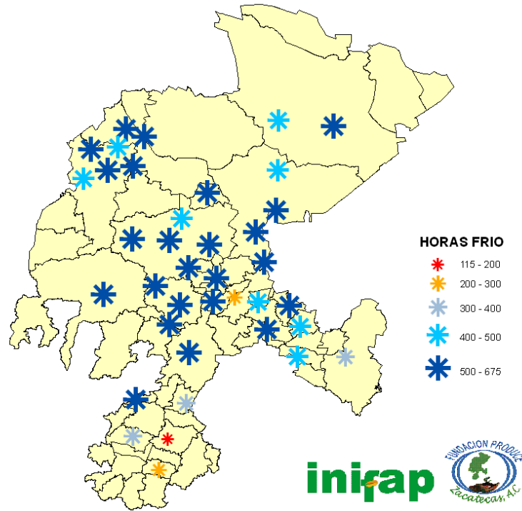
FIGURA 6. Horas frío acumuladas en los meses de noviembre a enero del 2016.
