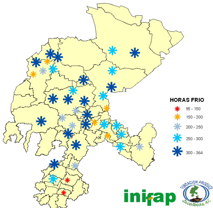
FIGURA 5. Horas frío acumuladas en el mes de enero del 2016.
