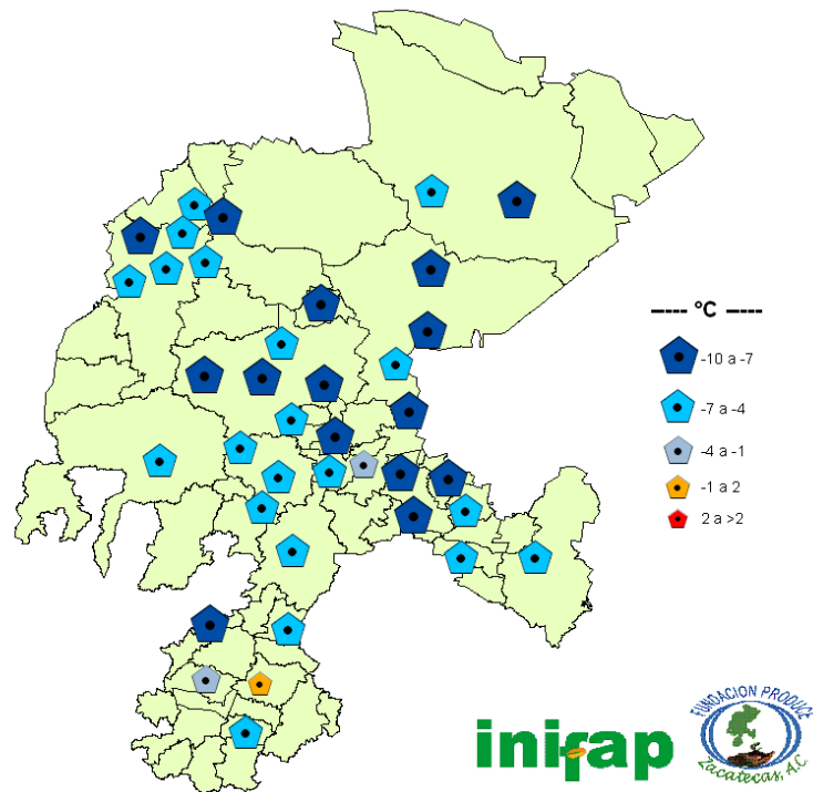
FIGURA 8. Valores mínimos de temperatura registrados en el mes de enero del 2016.
