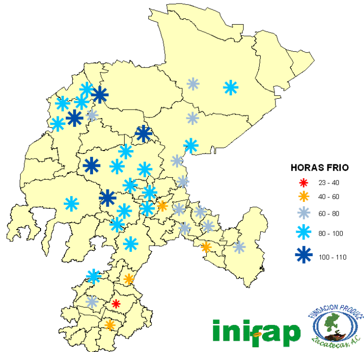
FIGURA 2. Horas frío acumuladas en la primera decena del mes de enero del 2016.
